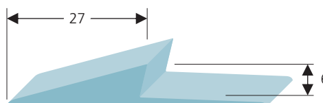
Tipo L 428 per soglie
