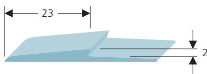
Tipo L 424 per soglie
