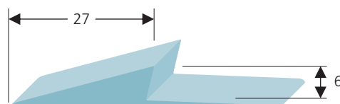
Typ L 428 Für Schmutzschleusen
