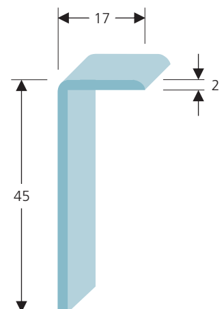
Typ L 308 Winkelprofil, passend zu TW 802/902
