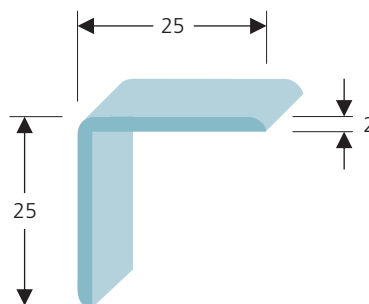
Typ L 301 Winkelprofil
