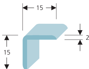
Typ L 300 Winkelprofil
